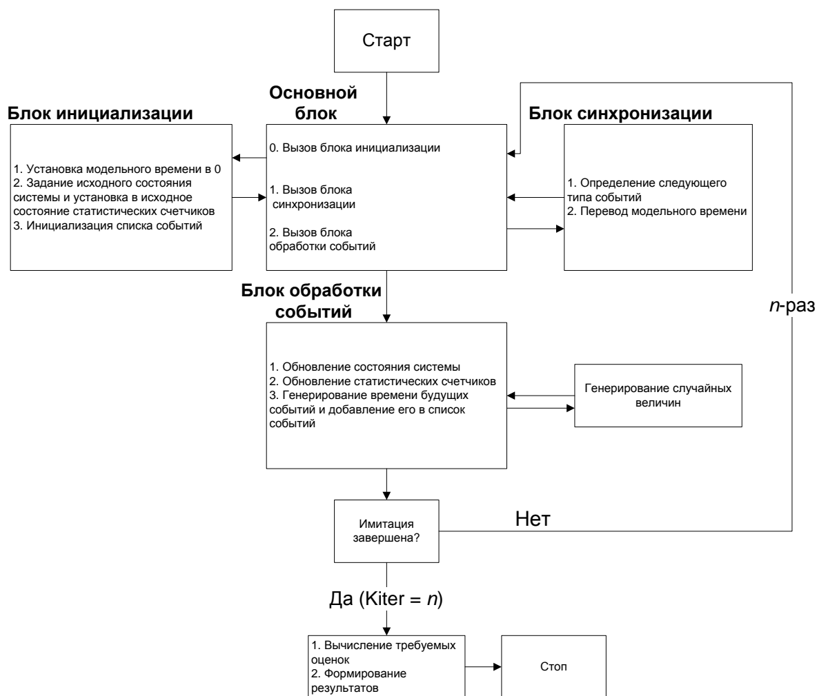
Рис. 1. Структурно-логическая схема дискретно-событийной имитационной модели
